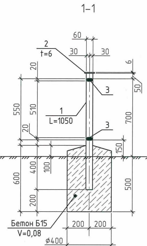
Спецификация элементов ограждения спортивной площадки
