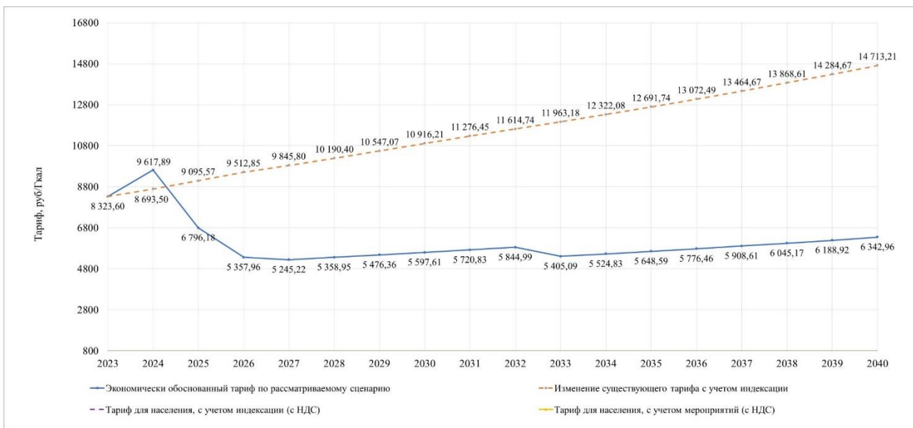
Рисунок 5. Результаты расчета ценовых последствий для потребителей ООО «АТГК» для сценария 2
