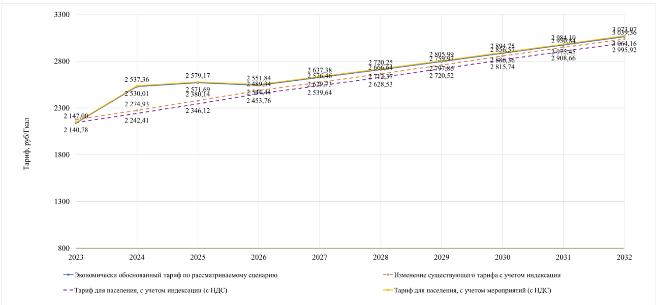
Рисунок 2. Результаты расчета ценовых последствий для потребителей ПАО «ТГК-2» для сценария 1)
